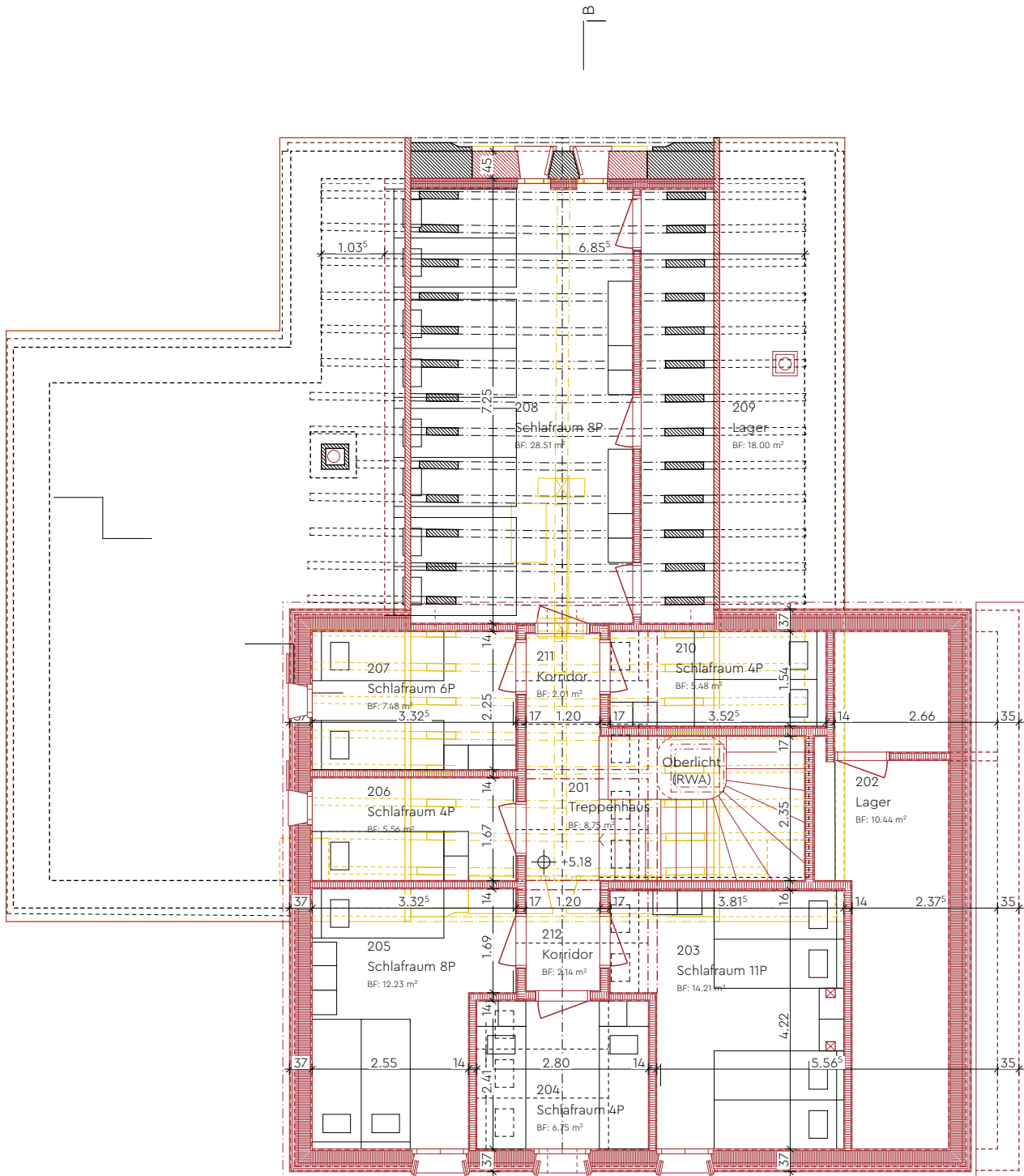
Dachgeschoss
