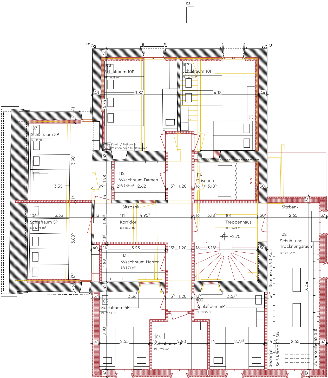
1. Obergeschoss
